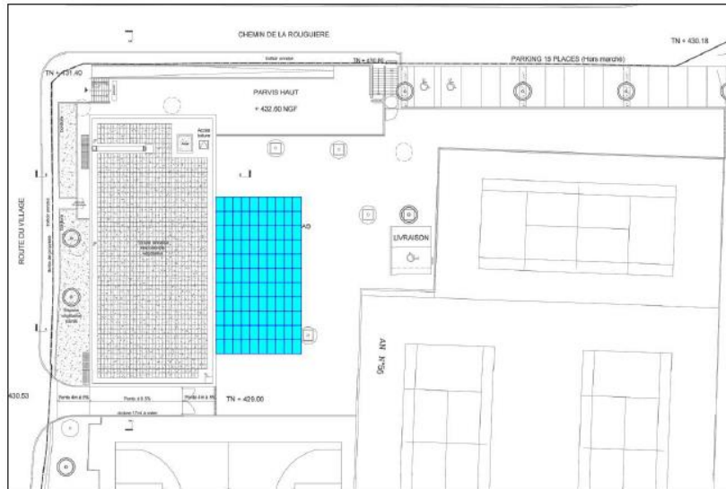
Implantation préau – 36 kWc
