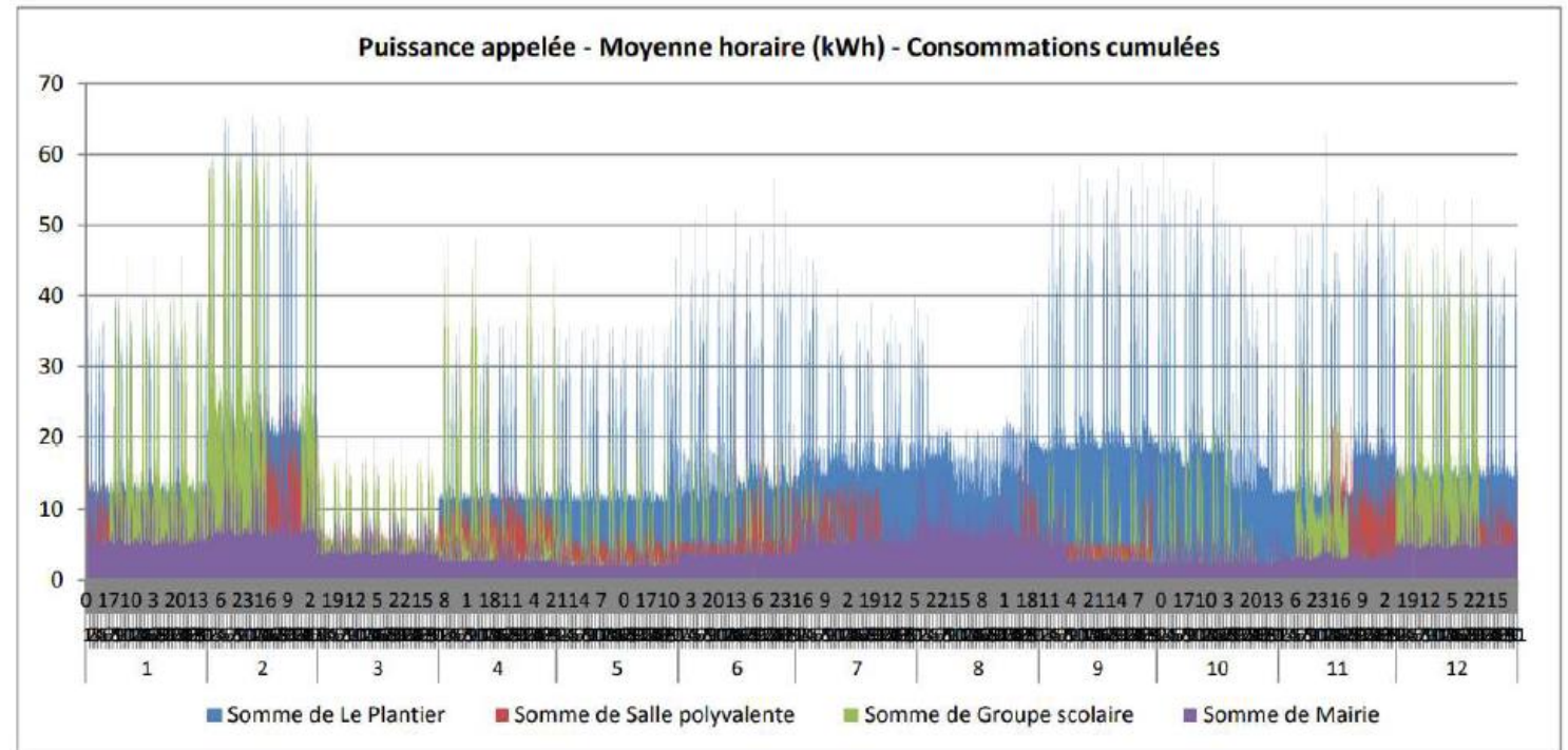
Profil de consommation des 4 sites
